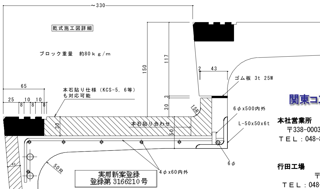
R形状のブロック接続部
