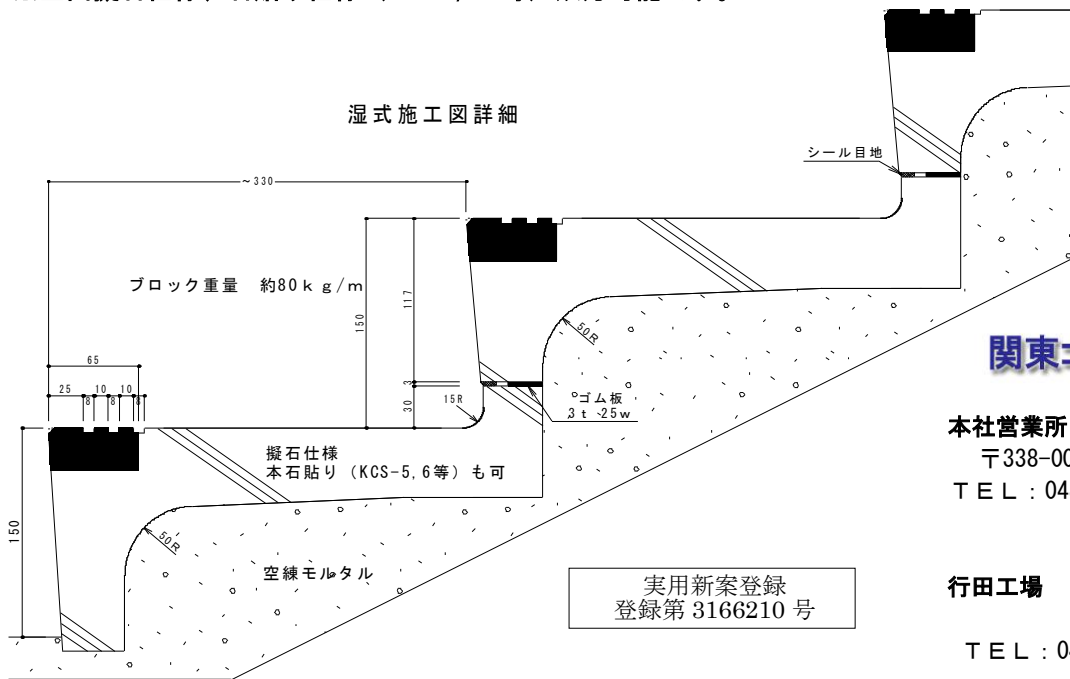
R形状のブロック接続部
